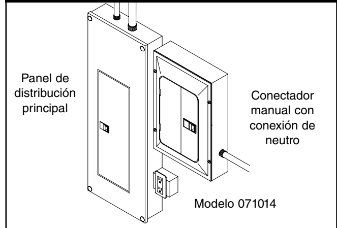
Figura 26 — Montaje habitual del conector
