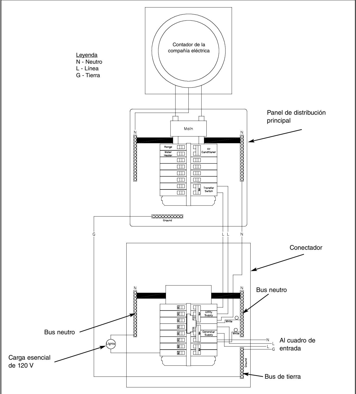
Figura 28 — Diagrama de instalación habitual del conector
